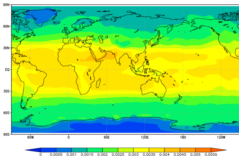
Рисунок 5.3.5 – Поле среднегодового прямого радиационного форсинга ( \text{Вт/м}^2 ) от возмущения концентрации метана в атмосфере, соответствующего минимальной оценке относительной величины выбросов метана ПАО «Газпром»
