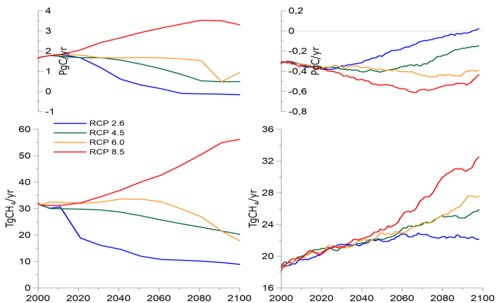
Рисунок 5.2.6в – Антропогенные (слева) и природные (справа) эмиссии CO 2 (вверху) и CH 4 (внизу) с территории Северной Америки
