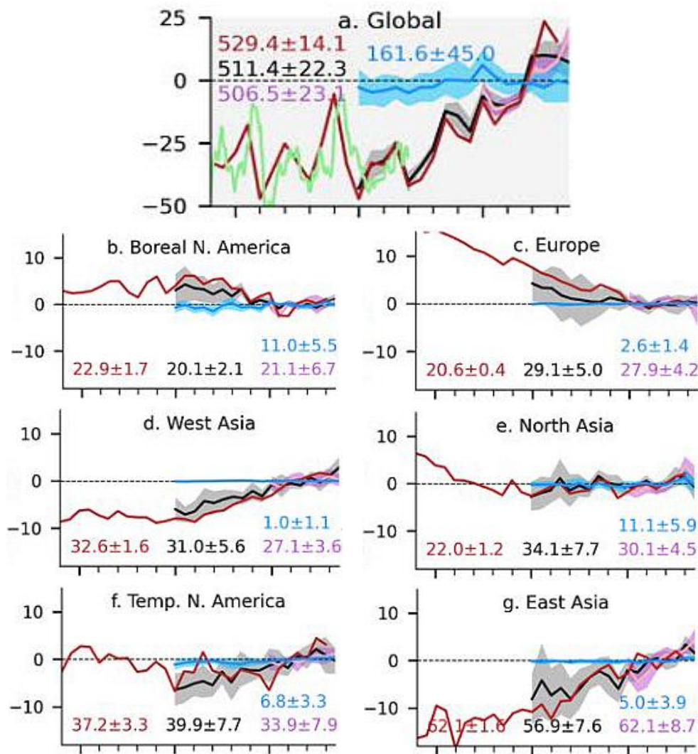
Рисунок 2.2.1 (воспроизведено по Cross-Chapter Box 5.2, Fig. 2 [37]) – Аномалии глобальных эмиссий метана и эмиссий из отдельных регионов Северного полушария за 1988–2017 гг. по данным ОД6 МГЭИК. Синим цветом обозначены эмиссии из влажных экосистем по модельным оценкам, другими цветами – суммарные эмиссии с поверхности на основании различных TD оценок. Средние многолетние значения за 2010–2016 годы (указаны отдельно на каждой панели), вычитались из среднегодовых временных рядов для расчета аномалий для каждого региона
