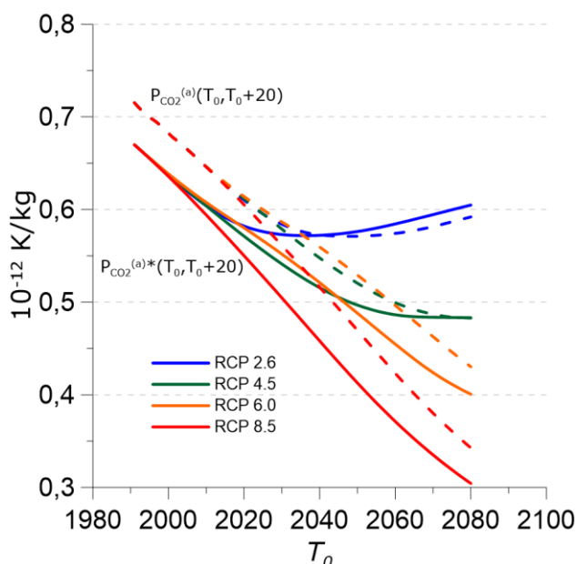
Рисунок 4.1.8 – Изменения 20-летних абсолютных потенциалов глобального изменения температуры P^{(a)} и P^{(a)*} (AGTP-20) для импульсной эмиссии углекислого газа в год T_0 при различных сценариях антропогенного воздействия
