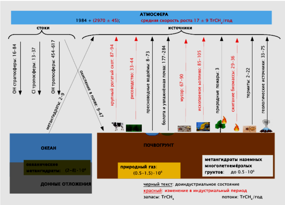
Рисунок 1.1.1 – Глобальный цикл метана (оценки для 2000-х гг.) согласно [1]
