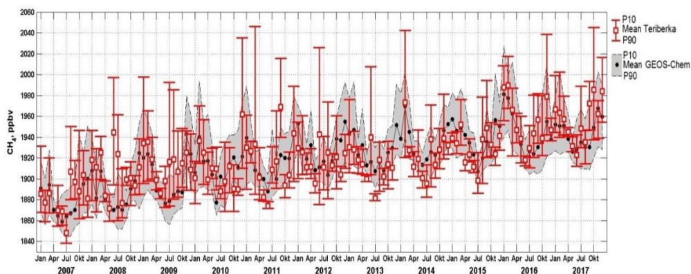
Рисунок 1.4.2 – Сравнение расчетов GEOS-Chem с наблюдениями приземной концентрации метана на станции Териберка
