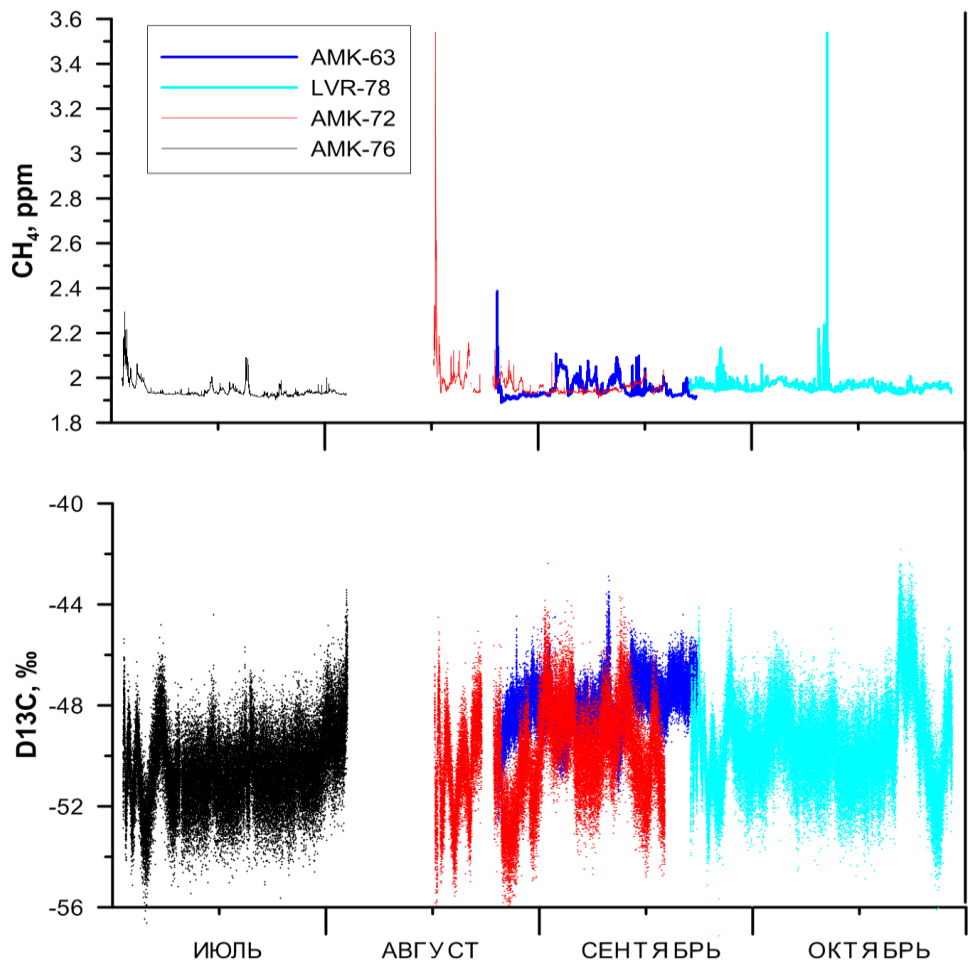
Рисунок 1.2.7 – Временные ряды \text{CH}_4 и \text{D13C} (G2132-i) в приповерхностном воздухе для экспедиций 2015, 2016, 2018 и 2020 гг.
