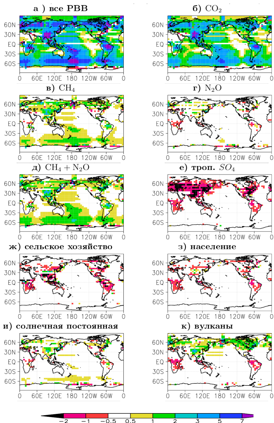
Рисунок 5.1.6 – Подобно рис. 5.1.5, но для годового количества осадков (см/год)
