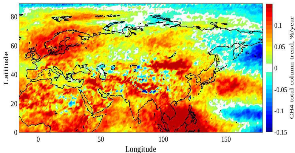
Рисунок 1.2.17 – Разница между трендами общего содержания метана по среднегодовым данным AIRS v6, разрешение 1 \times 1 градус, за период 2008–2019 и 2003–2008 гг.
