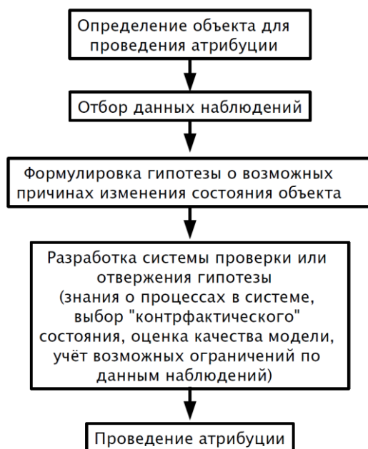
Рисунок 5.1.1 – Основные шаги построения атрибуции
