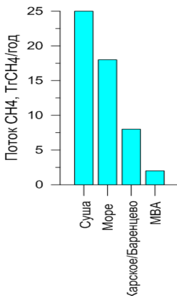
Рисунок 1.2.15 – Эмиссии метана по спутниковым оценкам для Арктики (выше 60^\circ \text{с.ш.} ) [56]
