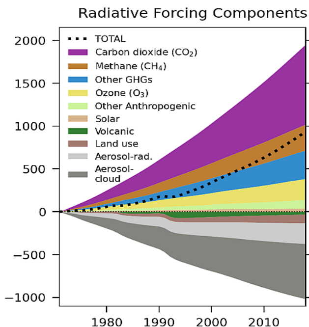
Рисунок 5.2.1 (Box 7.2 Fig.1e из [11]) – Накопление энергии ( 10^{21} Дж) в земной климатической системе, связанное с отдельными компонентами радиационного воздействия за индустриальный период по данным ОД6 МГЭИК
