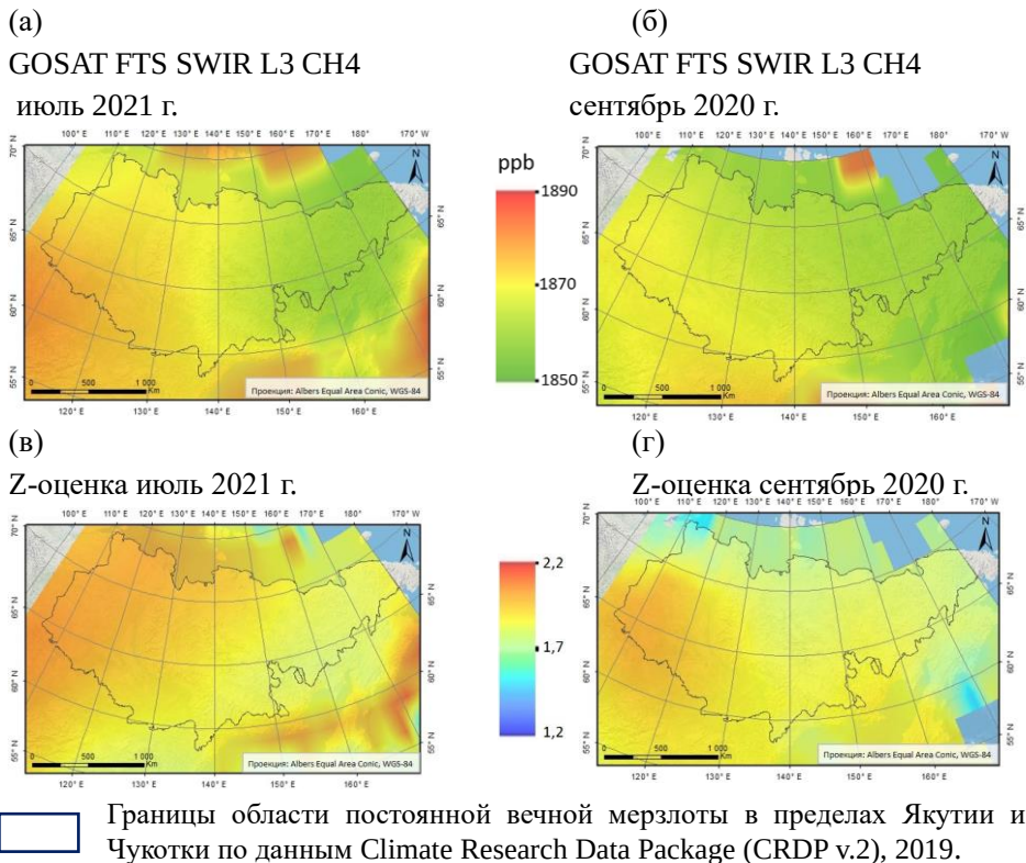
Рисунок 2.3.4 – Усредненные за месяц значения концентраций CH 4 в тропосфере по данным спутника GOSAT:
