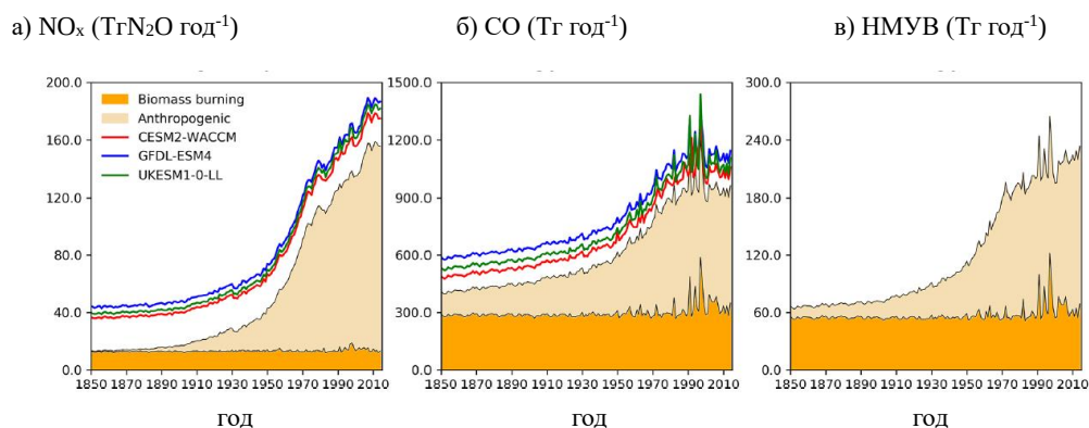
Рисунок 1.3.5 – Глобально осредненные предписанные эмиссии веществ в атмосферу, использованные в [17]. НМУВ – неметановые углеводороды, biomass burning – сжигание биомассы, anthropogenic – антропогенные. Остальные символы на легенде указывают на использованные модели.
