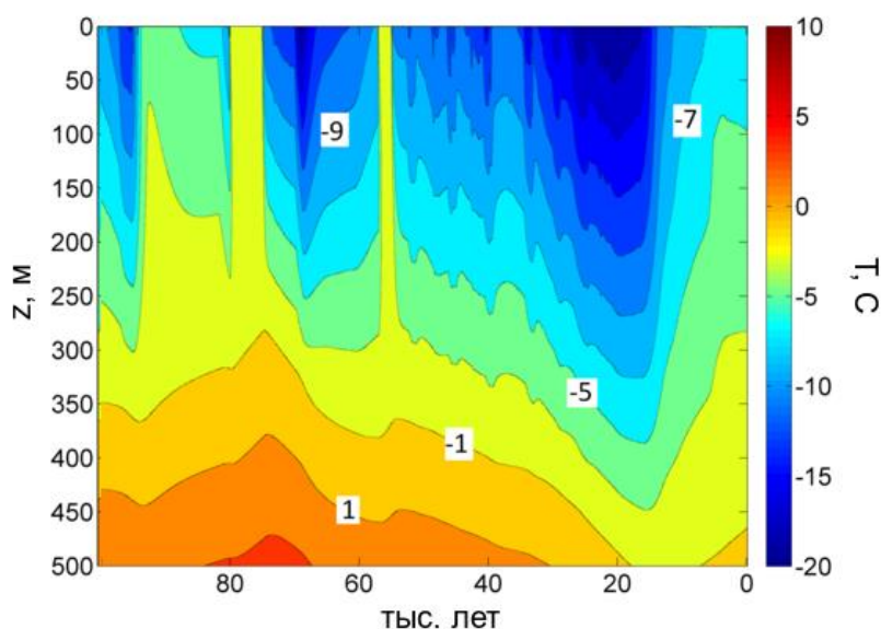
Рисунок 2.1.9 – Изменение среднегодовой температуры грунта за последние 100 тысяч лет в численном эксперименте G5
