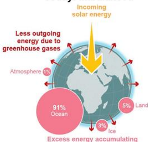
Рисунок 5.3.1 – Радиационный баланс земной системы в стабильном и нестабильном состояниях
