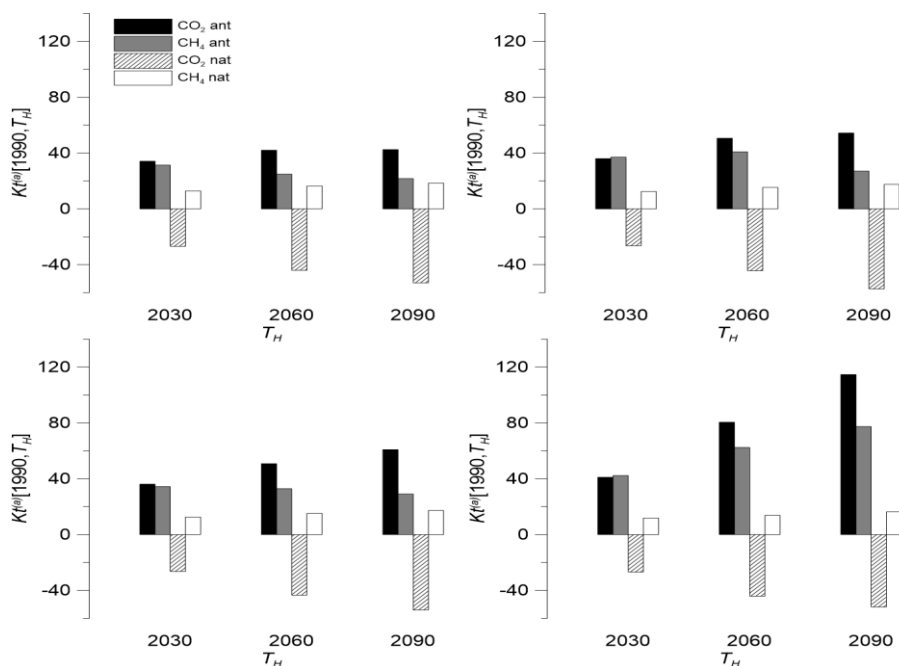
Рисунок 5.2.7а – Кумулятивный потенциал K_t [mK] антропогенных и природных эмиссий \text{CO}_2 и \text{CH}_4 с территории России на временных интервалах 1990–2030, 1990–2060 и 1990–2090 гг.
