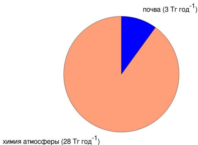
Рисунок 1.3.14 – Подобно рис. 1.3.11, но для данных территории России
