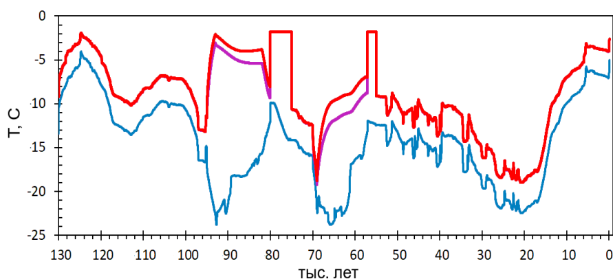
Рисунок 2.1.8 – Приповерхностная температура воздуха (синяя кривая), задаваемая в качестве верхнего граничного условия на подстилающей поверхности, в том числе на поверхности ледникового щита. Рассчитанные температуры поверхности грунта для интенсивности теплового потока 0,05 \text{Вт}/\text{м}^2 (фиолетовая кривая) и 0,07 \text{Вт}/\text{м}^2 (красная кривая)
