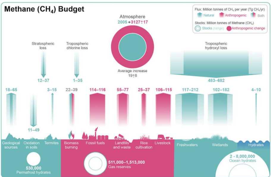
Рисунок 1.3.15 (рис. 5.14 из ОД6 МГЭИК [9]) – Глобальный бюджет метана для 2008–2017 гг. по данным ОД6 МГЭИК.
