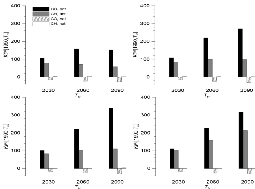
Рисунок 5.2.7б – Кумулятивный потенциал K_t [mK] антропогенных и природных эмиссий \text{CO}_2 и \text{CH}_4 с территории Китая на временных интервалах 1990–2030, 1990–2060 и 1990–2090 гг.
