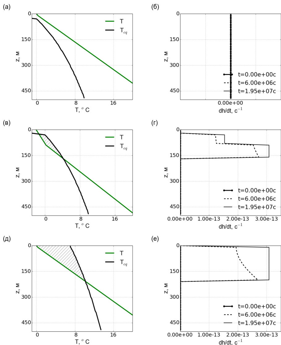
Рисунок 2.1.5 – Рассчитанные на основе профиля температуры грунта T и равновесной кривой метангидратов T_{eq} глубина z ЗС (а, в, д) и скорость гидратонакопления dh/dt (б, г, е) в различные моменты времени t ( 0,0 ; 6,0 \times 10^6 и 1,95 \times 10^7 с) с начала расчета для мощности ледника 200 м и температуры поверхности грунта 0^{\circ}\text{C} (а, б), мощности ледника 200 м и температуры поверхности грунта -2^{\circ}\text{C} (в, г) и мощности ледника 500 м и температуры поверхности грунта 0^{\circ}\text{C} (д, е). Значение теплового потока 0,05 \text{ Вт/м}^2 , глубина до газонасыщенного слоя 500 м
