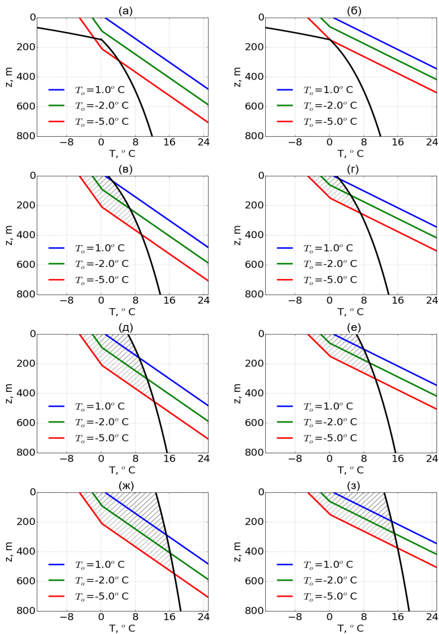
Рисунок 2.1.2 – Области формирования метангидратов (показаны штриховкой) для мощности ледникового щита 100 м (а, б), 300 м (в, г), 500 м (д, е) и 1000 м (ж, з), значениях теплового потока 0,05 Вт/м² (а, в, д, ж) и 0,07 Вт/м² (б, г, е, з) и температуре основания ледникового щита -5^\circ\text{C} , -2^\circ\text{C} и 1^\circ\text{C} (красная, зеленая и синяя линии, соответственно)
