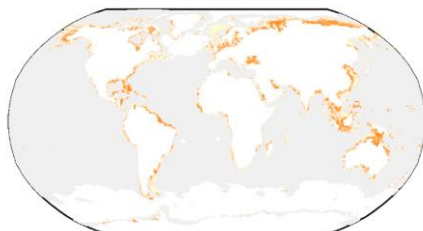
Рисунок 1.1.3 – Региональные годовые эмиссии метана ( \text{mgCH}_4 \text{ м}^{-2} \text{ сут.}^{-1} ) от разных источников для 2008-2017 гг. проекта «Глобальный бюджет метана». Воспроизведено по [24]
