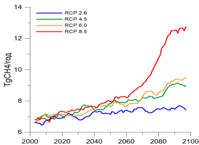
Рисунок 2.2.3 – Эмиссии метана из многолетнемерзлых болот России в XXI веке (7-летние скользящие средние) по расчетам с КМ ИФА РАН при различных сценариях антропогенного воздействия
