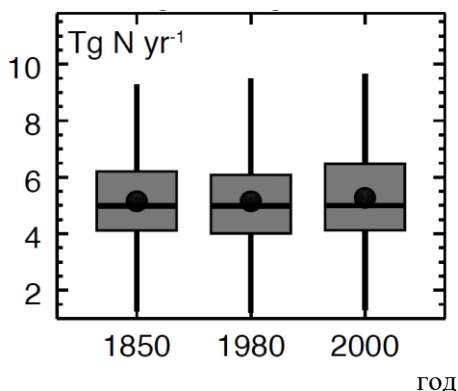
Рисунок 1.3.3 – Глобальные эмиссии неметановых углеводородов (а), CO (б), NO x (в) и вклад в последние эмиссии за счет молниевой активности (г), использованные при постановке численных экспериментов проекта ACCMIP.
