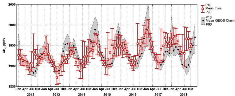
Рисунок 1.4.3 – Сравнение расчетов GEOS-Chem с наблюдениями приземной концентрации метана на станции Тикси
