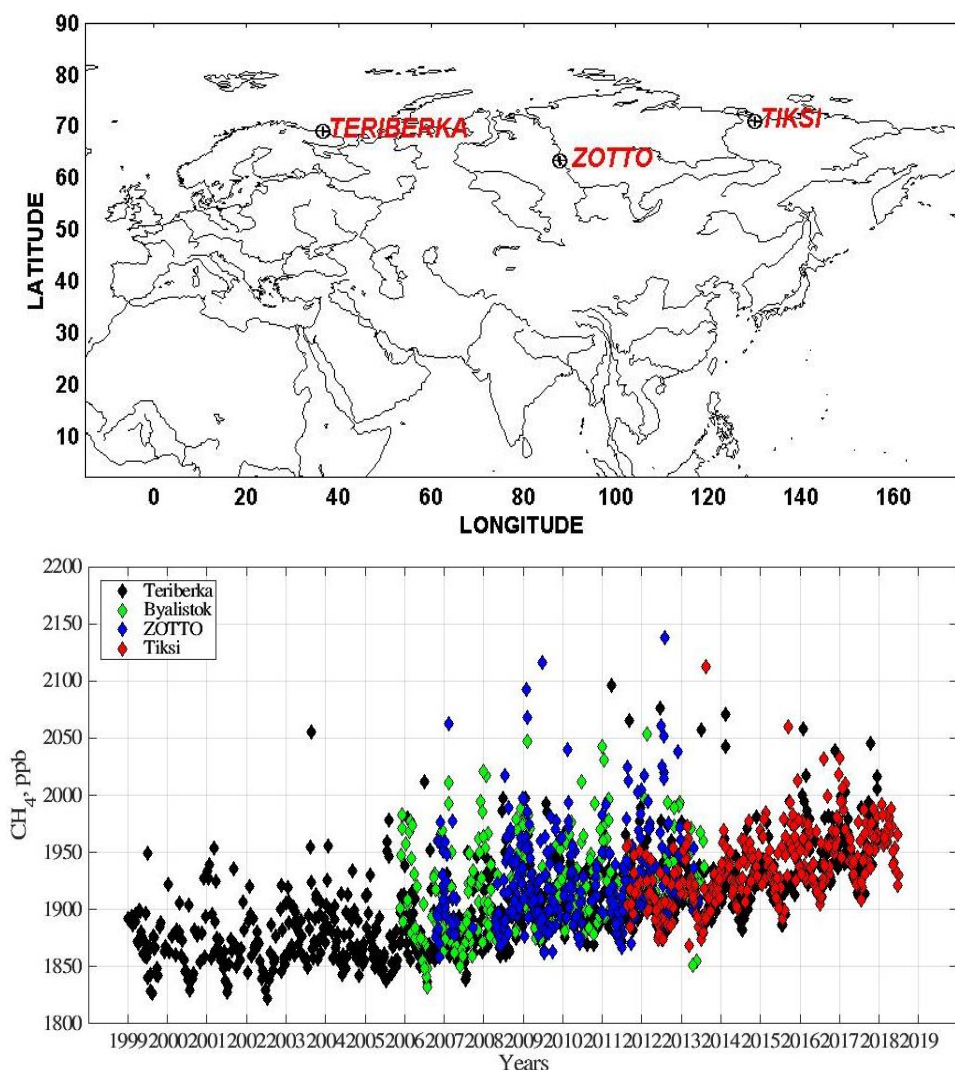
Рисунок 1.4.1 – Приземная концентрация метана по данным флаговых измерений на станциях Териберка, Белосток, ZOTTO и Тикси (см. карту сверху)
