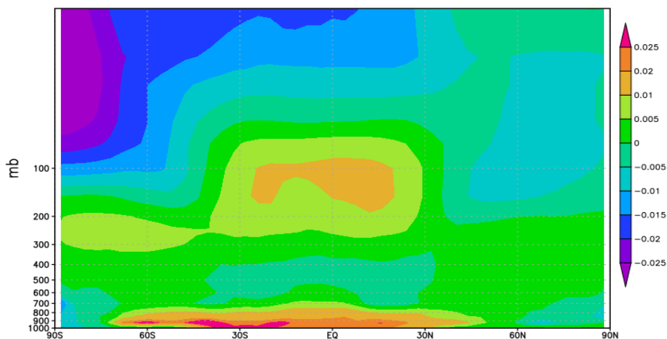
Рисунок 5.3.9 – Поле среднегодового среднезонального нагрева атмосферы (К/год) от возмущения концентрации метана в атмосфере, соответствующего максимальной оценке относительной величины выбросов метана ПАО «Газпром»
