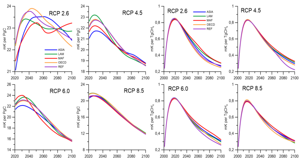
Рисунок 4.1.12 – «Климатическая стоимость» антропогенных эмиссий \text{CO}_2 (слева) и \text{CH}_4 (справа)
