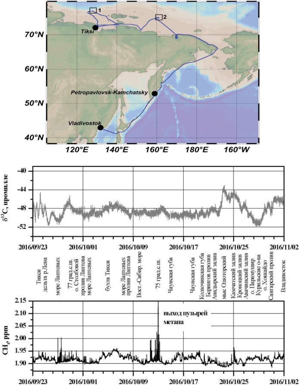
Рисунок 1.2.6 – Маршрут экспедиции и содержание изотопа δ 13 C CH 4 и концентрация метана в приводном воздухе по наблюдениям в рейсе № 78 НИС «Академик М.А. Лаврентьев» (2016 г.)
