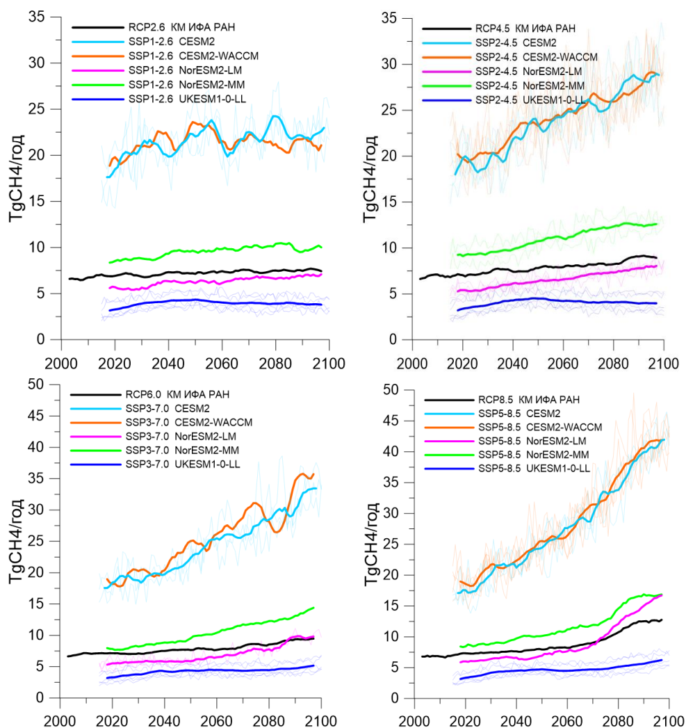
Рисунок 2.2.4 – Эмиссии метана из многолетнемерзлых болот России в XXI веке (7-летние скользящие средние) по расчетам с КМ ИФА РАН (черная линия) и моделей CMIP6 (цветные линии; при наличии нескольких реализаций одной модели толстой линией показано среднее, а тонкими сами реализации) при различных сценариях антропогенного воздействия
