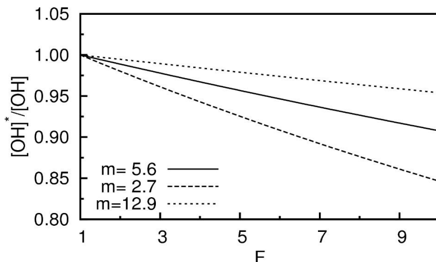
Рисунок 1.4.9 – Изменение среднеглобального содержания ОН в тропосфере ( [\text{OH}]^*/[\text{OH}] ) в зависимости от величины приращения антропогенных эмиссий молекулярного водорода F (=P_{\text{H}_2, \text{anthrop}}^*/P_{\text{H}_2, \text{anthrop}}) при различных величинах m=P_{\text{H}_2, \text{biog}}/P_{\text{H}_2, \text{anthrop}}
