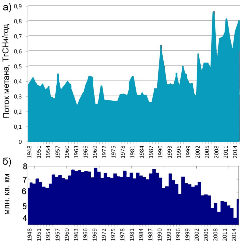
Рисунок 1.2.19 – (а) Поток метана в атмосферу из МВА (Тг CH 4 /год) и (б) рассчитанная площадь морского льда по расчетам [67]
