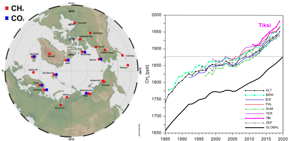
Рисунок 1.2.9 – Станции наблюдения \text{CO}_2 и \text{CH}_4 в высоких широтах Северного полушария (слева) и средняя годовая концентрация \text{CH}_4 на полярных станциях. ALT – Аллерт, BRW – Барроу, ICE – Хаймей, PAL – Паллас, SUM – Саммит, TER – Териберка, TIK – Тикси, ZEP – Цеппелин [NOAA/ESRL, WMO World Data Centre for Greenhouse Gases], GLOBAL – глобальная по данным NOAA [www.esrl.noaa.gov/gmd/ccgg/trends_ch4]
