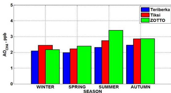
Рисунок 1.4.7 – Сводная диаграмма величин AO_{CH_4} на эмиссии метана от антропогенных (а) и биогенных (б) источников и горения биомассы (в) для станций Териберка, Тикси и ZOTTO. Приведены средние значения для всех сезонов 2007–2018 гг.
