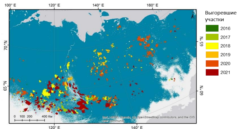
Рисунок 2.3.1 – Границы выгоревших участков в зоне сплошного распространения вечномерзлых пород (показано синим фоновым цветом) в период с 2016 по 2021, восстановленные по спутниковым данным VIIRS ActiveFire
