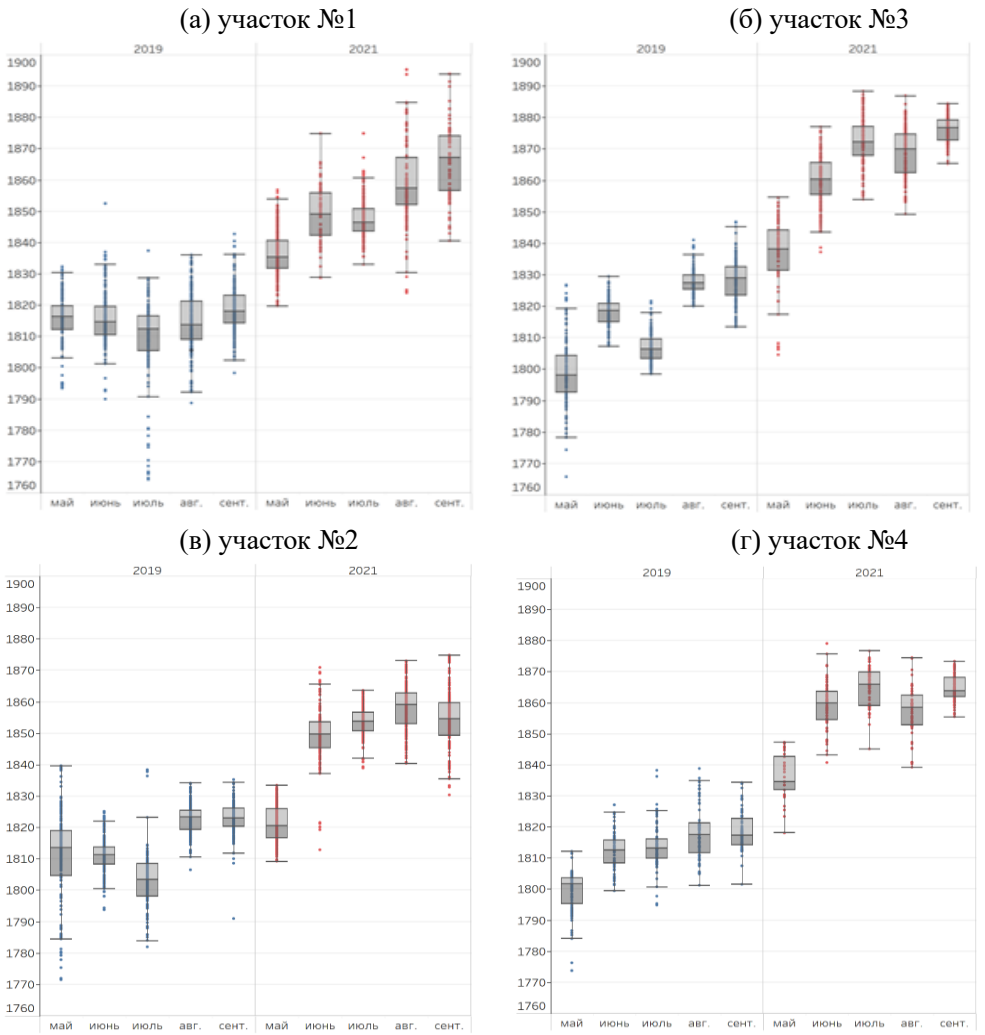
Рисунок 2.3.7 – Динамика концентраций метана над горящими в допозарный(2019) и постпожарный (2021) годы по спутниковым данным TROPOMI
