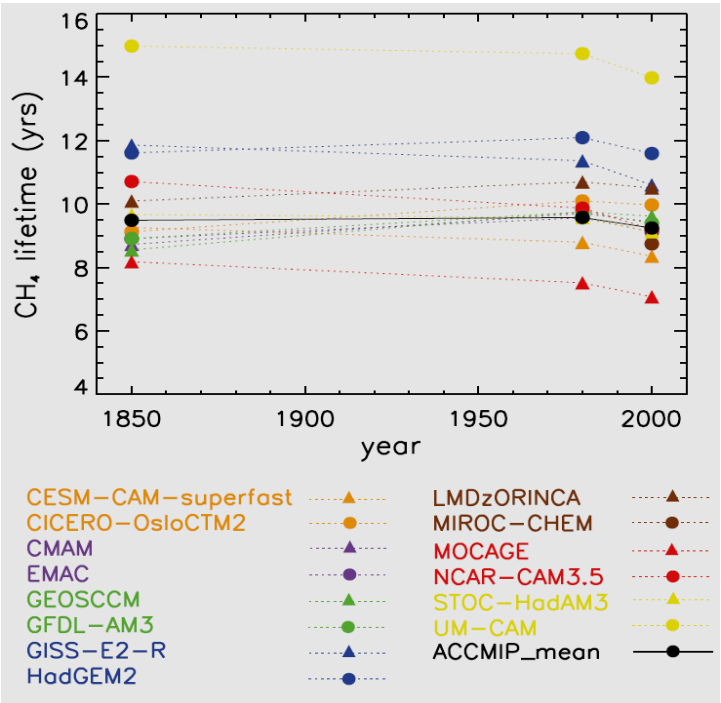
Рисунок 1.3.7 – Зависимость времени жизни метана в атмосфере от времени по результатам проекта ACCMIP (воспроизведено по [12]). На легенде указаны модели, участвующие в проекте за исключением «ACCMIP_mean», которое обозначает среднее по ансамблю значение. Перевод остальных терминов: CH 4 lifetime (yrs) – время жизни метана в атмосфере (годы); year – год
