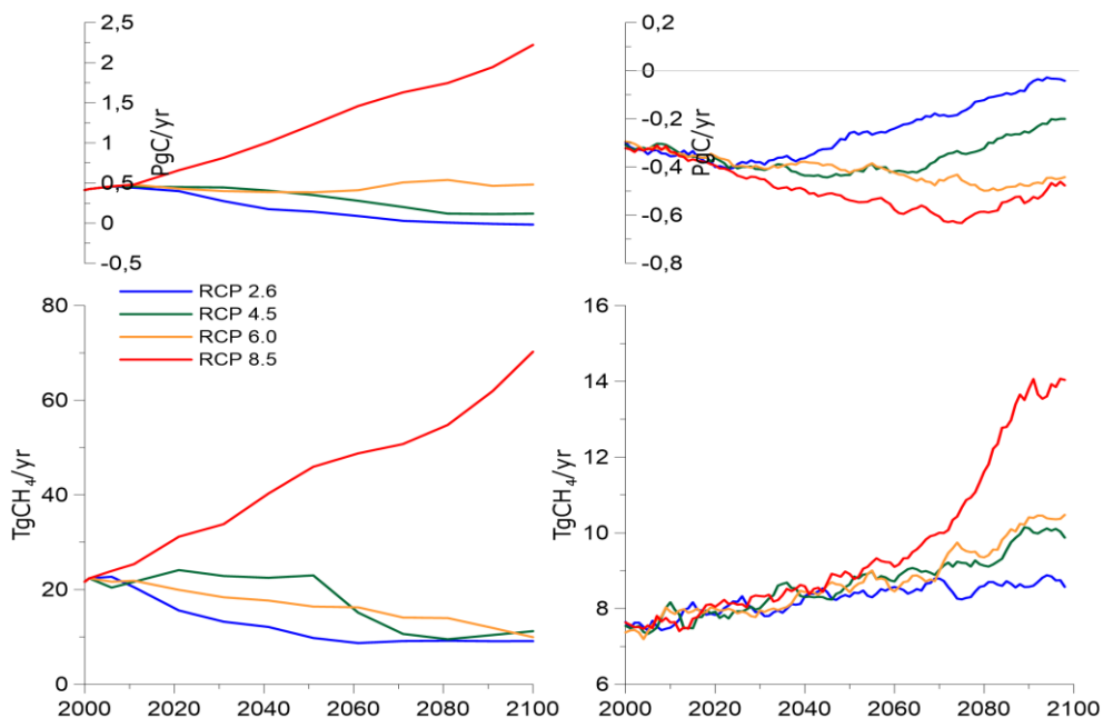
Рисунок 5.2.6а – Антропогенные (слева) и природные (справа) эмиссии \text{CO}_2 (вверху) и \text{CH}_4 (внизу) с территории России
