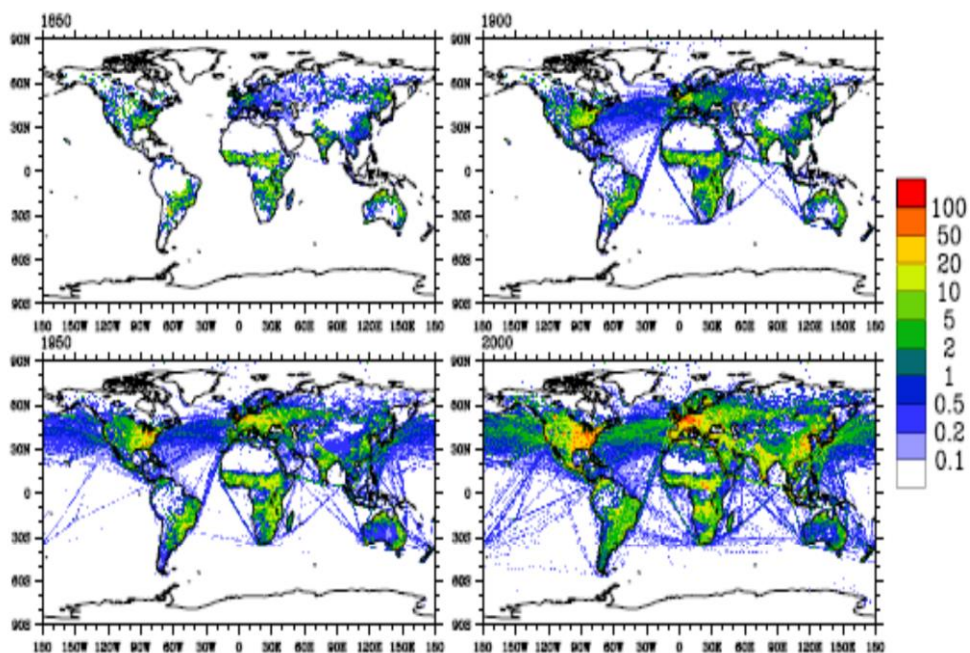
Рисунок 1.3.4 – Пространственное распределение не связанных с молниевой активностью эмиссий \text{NO}_x для временных срезов проекта ACCMIP
