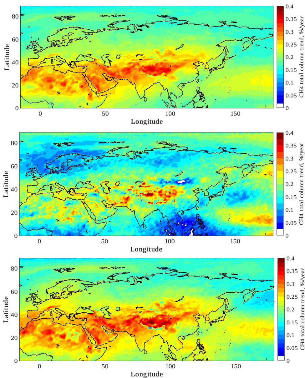
Рисунок 1.2.16 – Тренды общего содержания метана по среднегодовым данным AIRS v6, разрешение 1×1 градус, для 2003–2019 (а), для 2003–2008 (б) и для 2008–2019 гг. (в)
