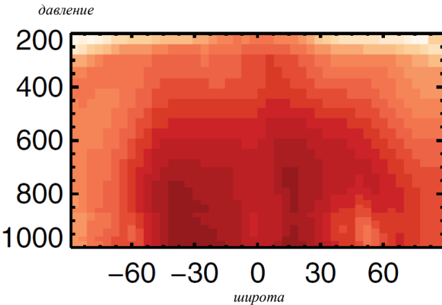
Рисунок 1.3.8 – Пространственно-временные вариации параметра p для обратной связи \tau_{CH4} = \tau_{CH4}(q_{CH4}) . Воспроизведено по [20]
