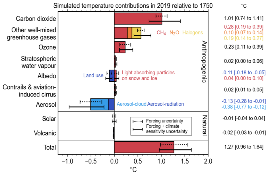
Рисунок 5.2.3 (Fig. 7.7 из [11]) – Рассчитанное изменение GSAT [°C] в 2019 году по отношению к 1750 году, связанное с основными антропогенными и природными факторами воздействия по данным ОД6 МГЭИК. Также приведены (5–95%) доверительные интервалы оценок, при этом пунктиром указан разброс, связанный только с неопределенностью радиационного форсинга (см. рис. 5.2.2), а сплошными линиями – итоговый разброс с учетом неопределенности климатического отклика
