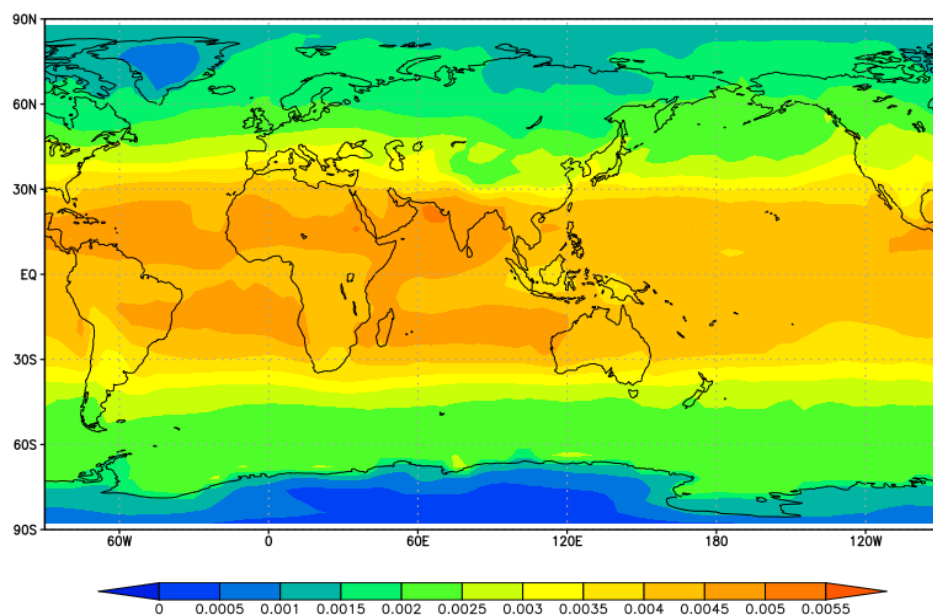
Рисунок 5.3.6 – Поле среднегодового прямого радиационного форсинга ( \text{Вт/м}^2 ) от возмущения концентрации метана в атмосфере, соответствующего максимальной оценке относительной величины выбросов ПАО «Газпром»
