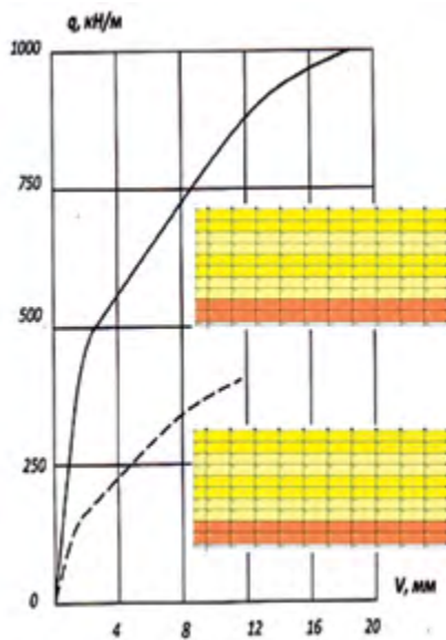
Рис. 56. Верхний график прогибов и трещинообразования – из ВБ, нижний – из обычного бетона.
