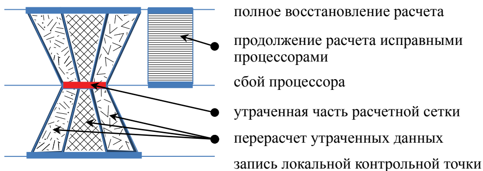
Рис. 1. Новый метод локального парирования ошибок вычислительных узлов суперкомпьютера
