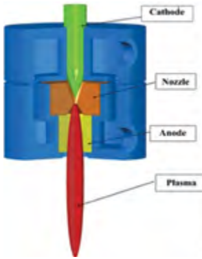
Плазматрон для синтеза графенов
