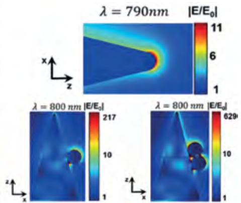
Распределение напряженности электрического поля в изолированной наночастице на резонансной длине волны
