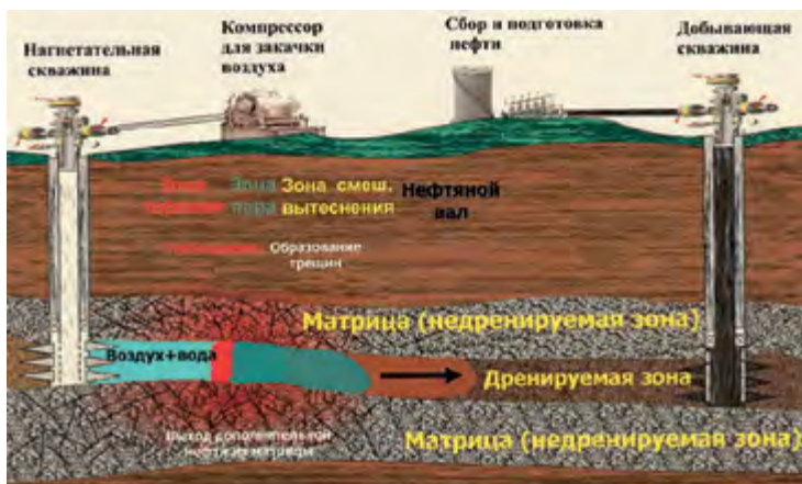
Рис. 19. Метод термогазового воздействия для повышения нефтеотдачи.
