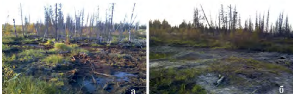
Рис. 31. Очистка нефтезагрязненных грунтов при низких положительных температурах: а - нефтезагрязненный участок до рекультивации (Пуровский район, Ямало-Ненецкий автономный округ, Тюменская область.); б - тот же участок после рекультивации с применением биопрепарата на основе штамма бактерий Pseudomonas turukhanskensis .
