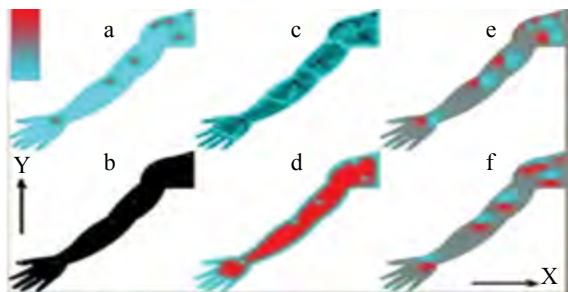
Рис. 4. Результаты вычислительных экспериментов по многоточечному тепловому воздействию на образец сложной геометрической формы.
