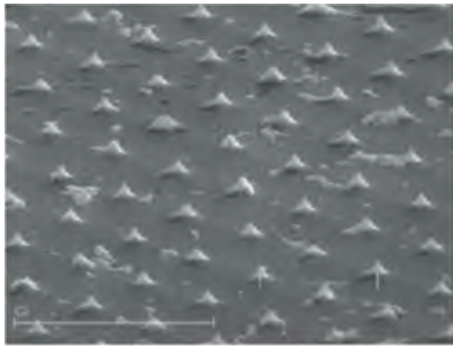
ГКР-сенсор: площадь поверхности 2x2 мм, период, диагональный период 2.12 мкм, высота 0.3-0.7 мкм, угол при вершине 30°, радиус кривизны \pm 10 нм. Радиус наночастиц золота (56 ± 1) нм
