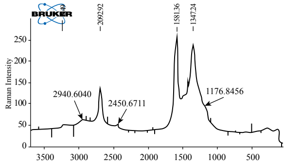
Рамановский спектр гидрированного графена
