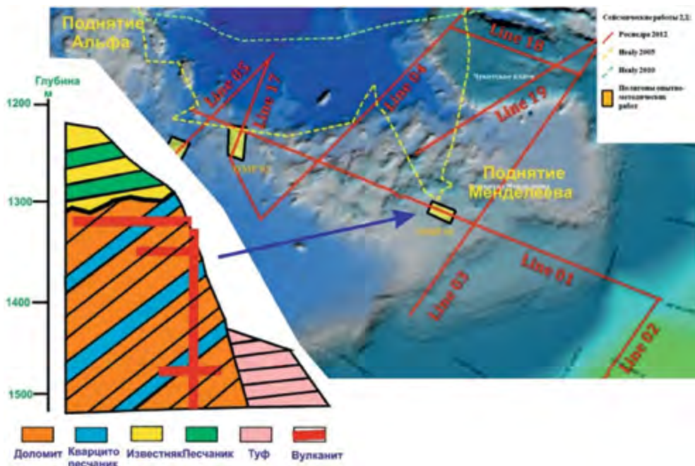
Рис. 38. Разрез акустического фундамента юго-западной части поднятия Менделеева
