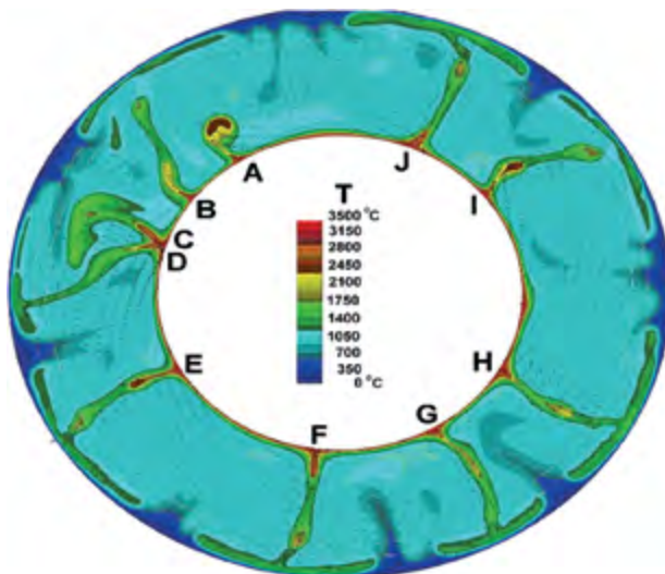
Рис. 37. Рассчитанное поле температуры и скорости течений в экваториальном сечении мантии Земли.
