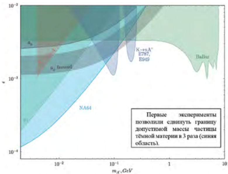
Рис. 11. Ограничения области существования тёмных фотонов в зависимости от их массы на 95% уровне достоверности, полученные в эксперименте NA64 и в других экспериментах: ВаBar и E787+E949.
