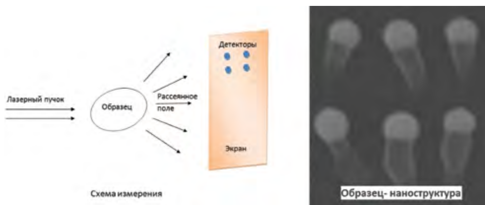
Рис. 3. Схема измерения (слева) и наноструктура (справа).
