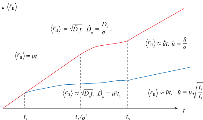
Рис. 22. Среднее смещение частиц примеси в статистически однородной резко контрастной среде при наличии (—) и в отсутствие (—) коллоидов.
