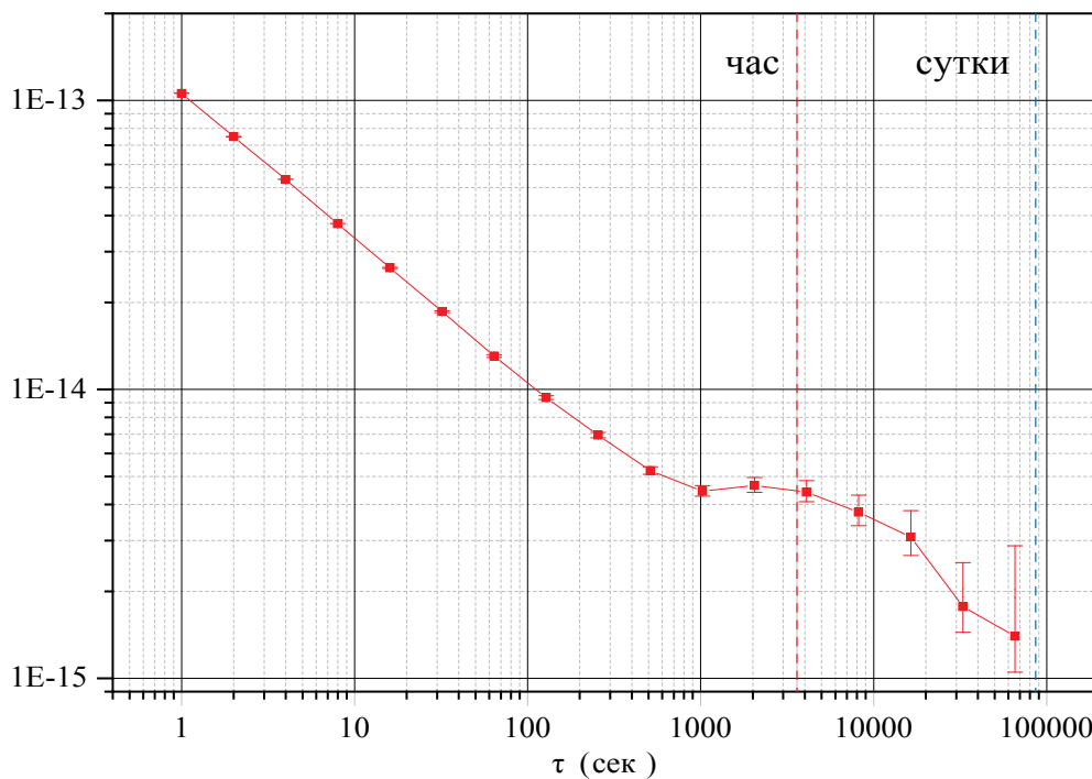
Рис. 14. Параметр Аллана для фемтосекундных оптических часов.
