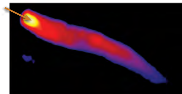
Рис. 6. Открытие экстремальной яркости ядра квазара 3C273.
