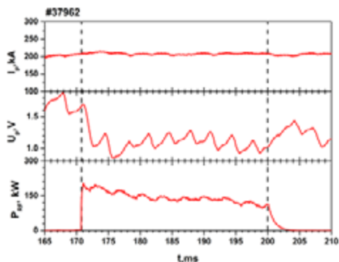
Рис. 15. Эффект замещения индукционного тока током увлечения, наблюдаемый по характерному снижению напряжения на обходе плазменного шнура U_p при неизменном полном токе плазмы I_p
