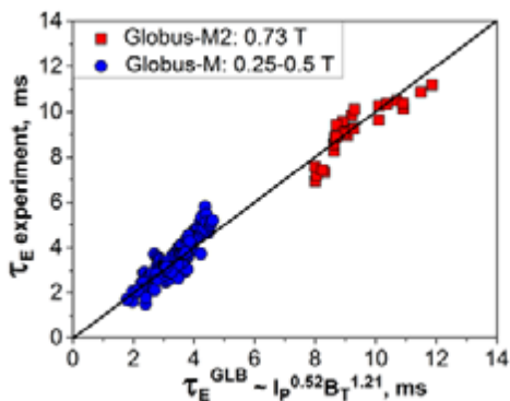
Рис. 14. Сравнение времени удержания энергии при низких и высоких магнитных полях
