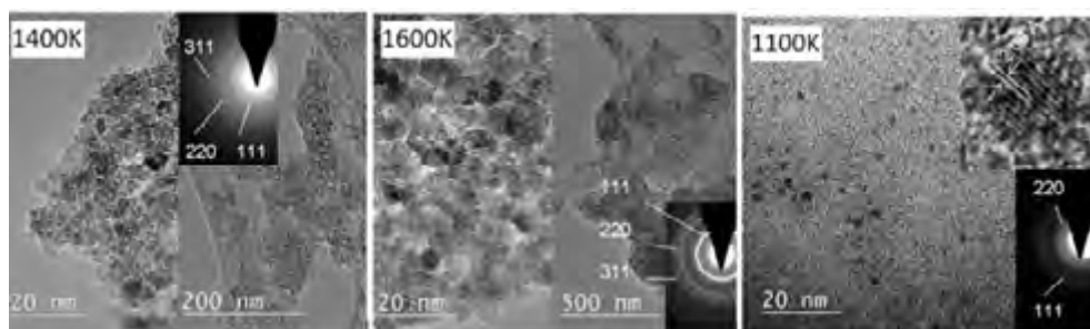
Рис. 16. Синтез наноалмазов из бромированного адамантана C10H14Br при 8 ГПа, время синтеза 120 с.
