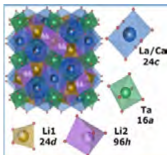
Рис. 23. Кристаллическая решётка литиевых гранатов на основе оксидов Nb, Hf, Ta, как например, изображённого кубического граната \text{Li}_{5+x} \text{Ca}_x \text{La}_{3-x} \text{Ta}_2 \text{O}_{12} является отличной оптической матрицей для ионов РЗЭ
