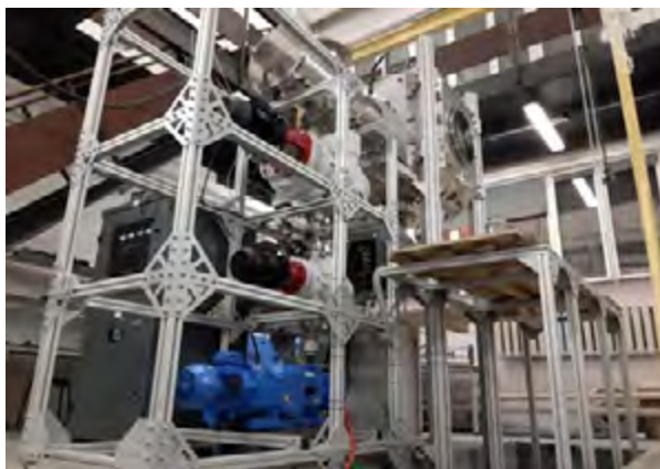
Рис. 21. Стенд «Испаритель»
