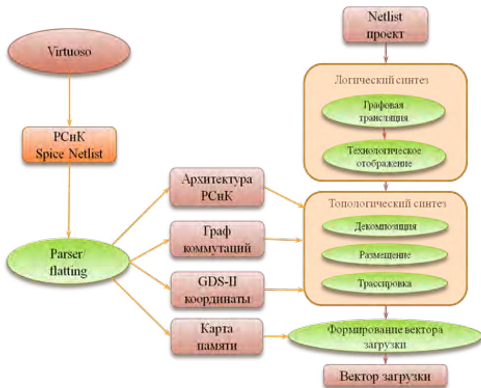
Рис. 6. Блок-схема маршрута проектирования полукастомных схем на базе РСнК
