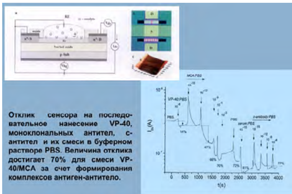
Рис. 51. Нанотранзисторные сенсоры для детектирования вирусов
