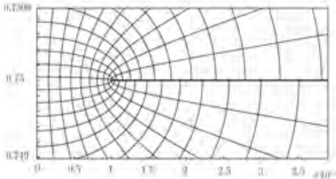
Рис. 3. Пример решения проблемы «кроудинга» в области с узким перешейком: (a) конформная сетка во всей области, (b) сетка вблизи узкого перешейка
