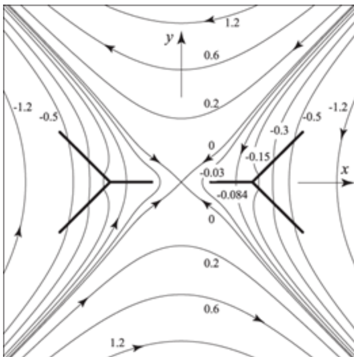
Рис. 2. Магнитное поле вблизи распадающегося токового слоя в области пересоединения
