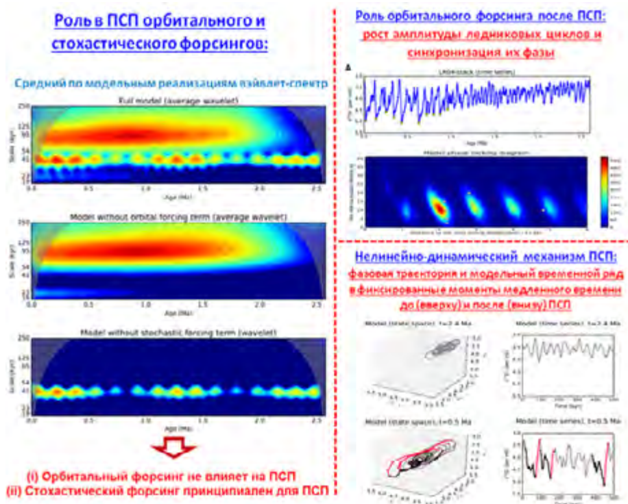
Рис. 34. Эмпирическое моделирование климата прошлого
