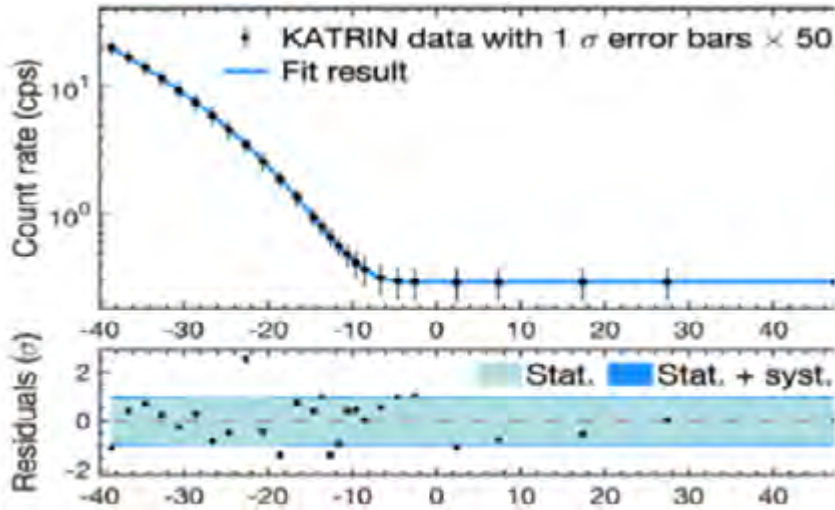
Рис. 20. Спектр электронов распада молекулярного трития НТ вблизи граничной точки, измеренный в первом сеансе КАТРИН. Вверху: абсолютные единицы; внизу: отклонения от теоретического спектра, деленные на экспериментальные ошибки
