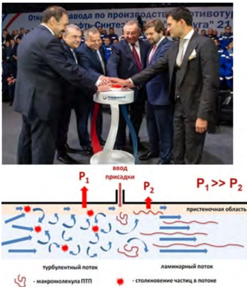
Рис. 27. Запуск нового завода и технология производства противотурбулентных присадок. Протяженные макромолекулы полимера ( M > 1 млн. Да), добавленные в поток, ориентируются вдоль движения жидкости и сглаживают высокочастотные пульсации давления (Эффект Томса). Эффективность использования полимера проявляется при концентрациях 1 ррт. Применение ПТП позволяет существенно понизить турбулентность в потоке перекачиваемой жидкости, уменьшить гидравлическое сопротивление и энергозатраты, увеличить пропускную способность трубопровода на 20% и выше, а также повысить срок эксплуатации оборудования
