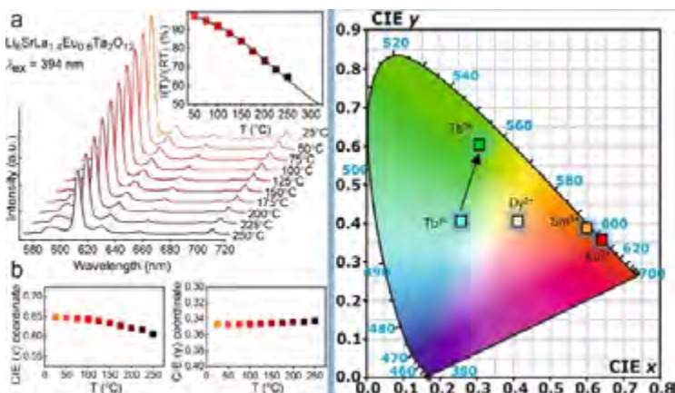
Рис. 24. Синтезирована новая группа люминофоров на основе литиевых гранатов. Введение диспрозия вызывает люминесценцию с близкими к белому цвету цветовыми координатами.
