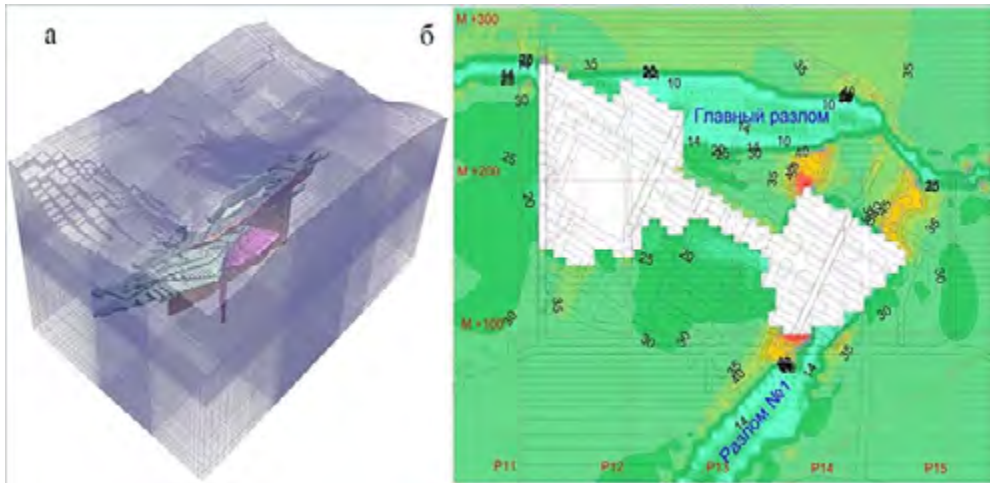
Рис. 31. а – 3D вид разработанной численной модели; б – распределение напряжений отах на гор. +120 м при фактическом состоянии горных работ на окт. 2019 г.
