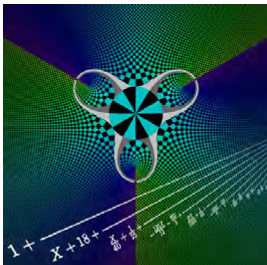
Рис.1. Эллиптическая кривая и ассоциированная с ней функциональная непрерывная дробь
