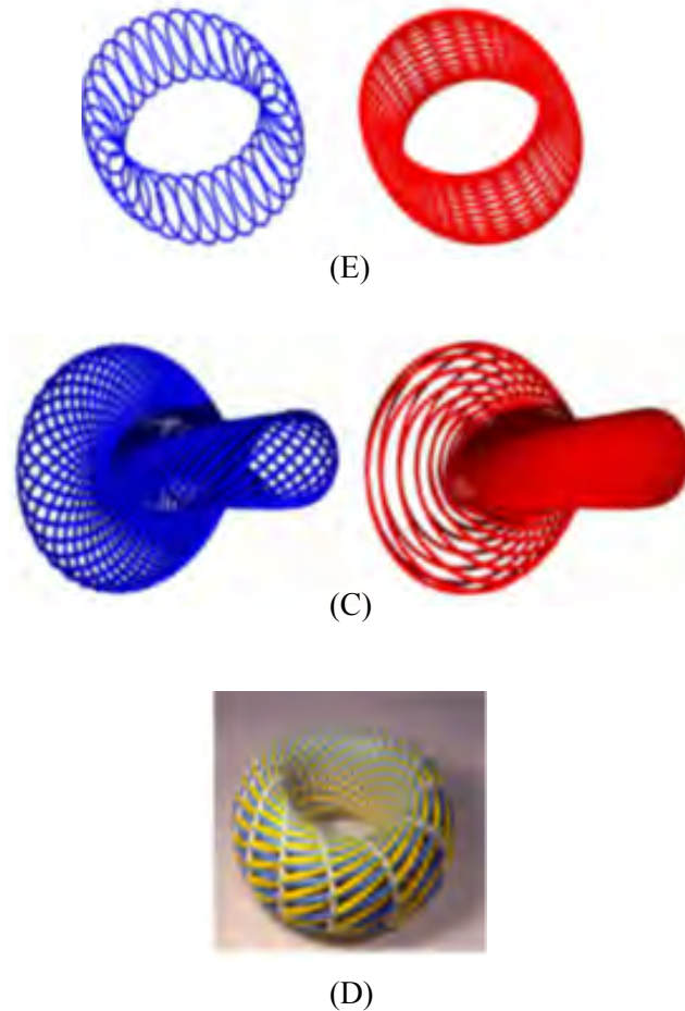
Рис. 4. Евкойдовы (E) и клиффордовы (C) трансляционные поверхности, и циклида Дарбу (D)
