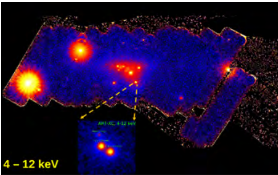
Рис. 8. Рентгеновское изображение центральной области Галактики в диапазоне 4–12 кэВ, полученное телескопом ART-XC
