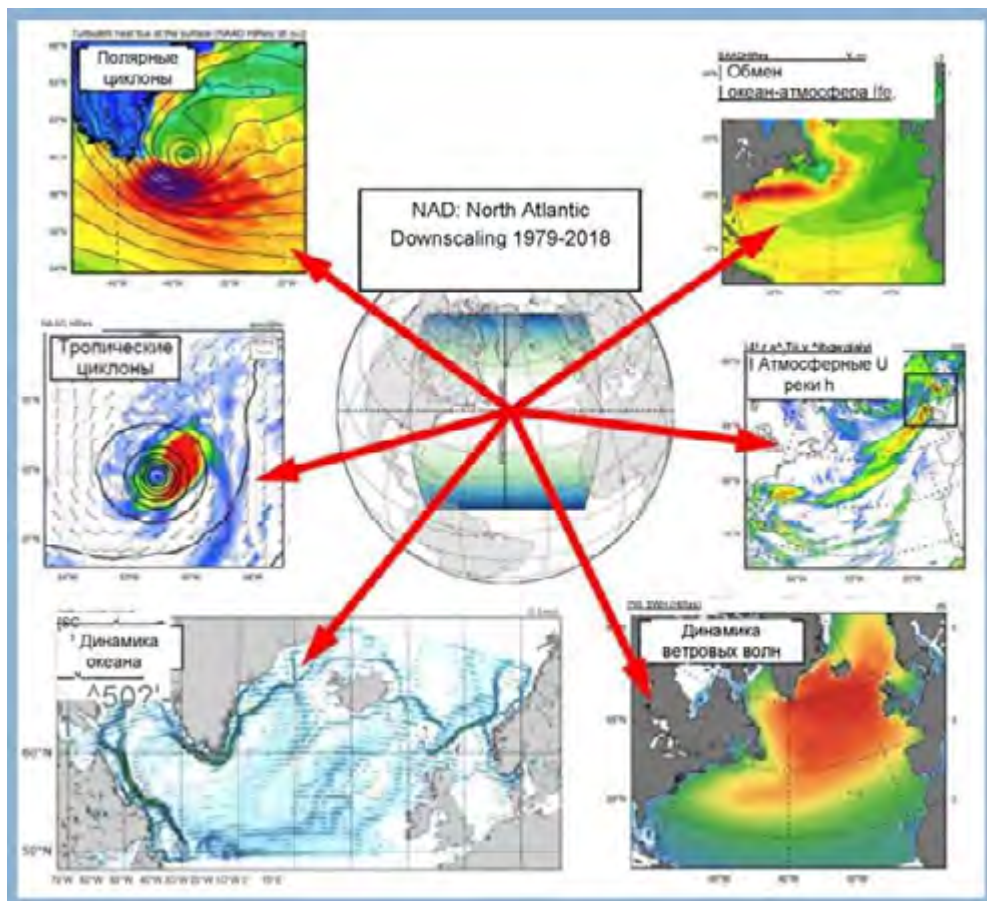
Рис. 32. Модель динамики атмосферы над Северной Атлантикой
