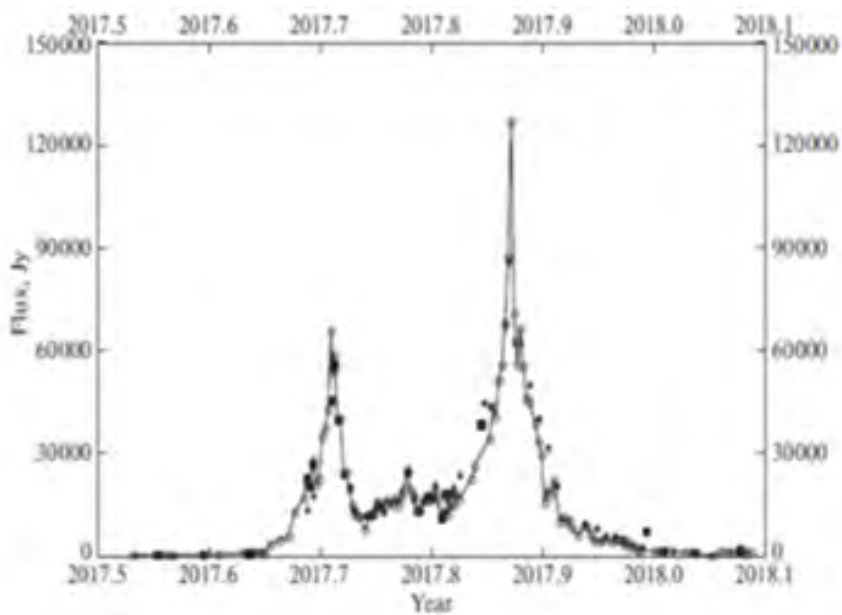
Рис. 11. Кривая плотности потока излучения во время вспышки
