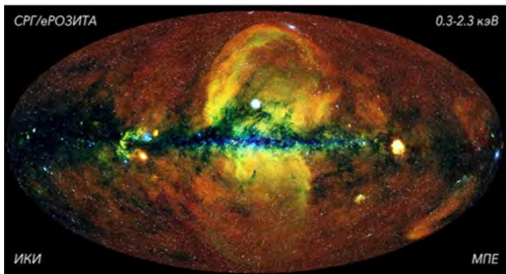
Рис. 10. Полная карта звездного неба в рентгеновских лучах, полученная в результате полугодовых наблюдений на «Спектр-РГ»
