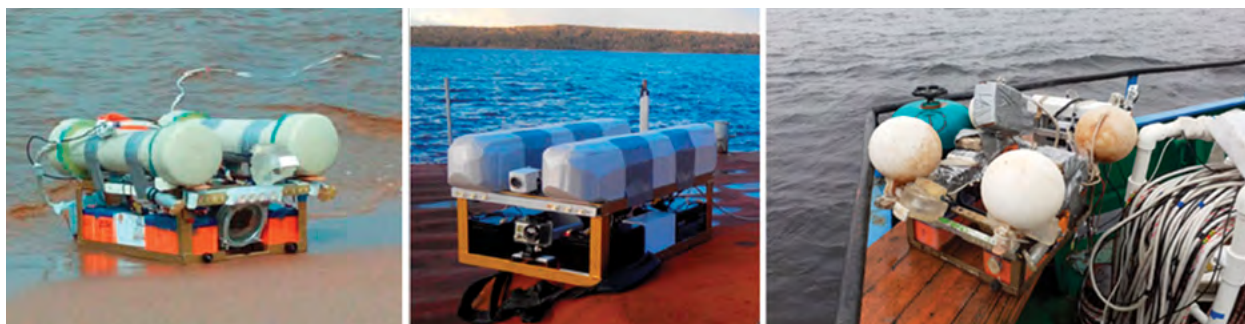
Рис. 5.1. Телеуправляемый необитаемый подводный аппарат Limnoscout-230 в различных модификациях 2018–2020 гг.
