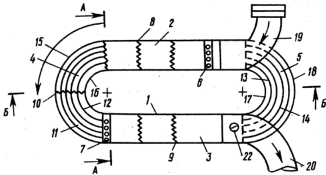
Рис. 12.1. Схематическое изображение установки «Аэрогидроканал»
