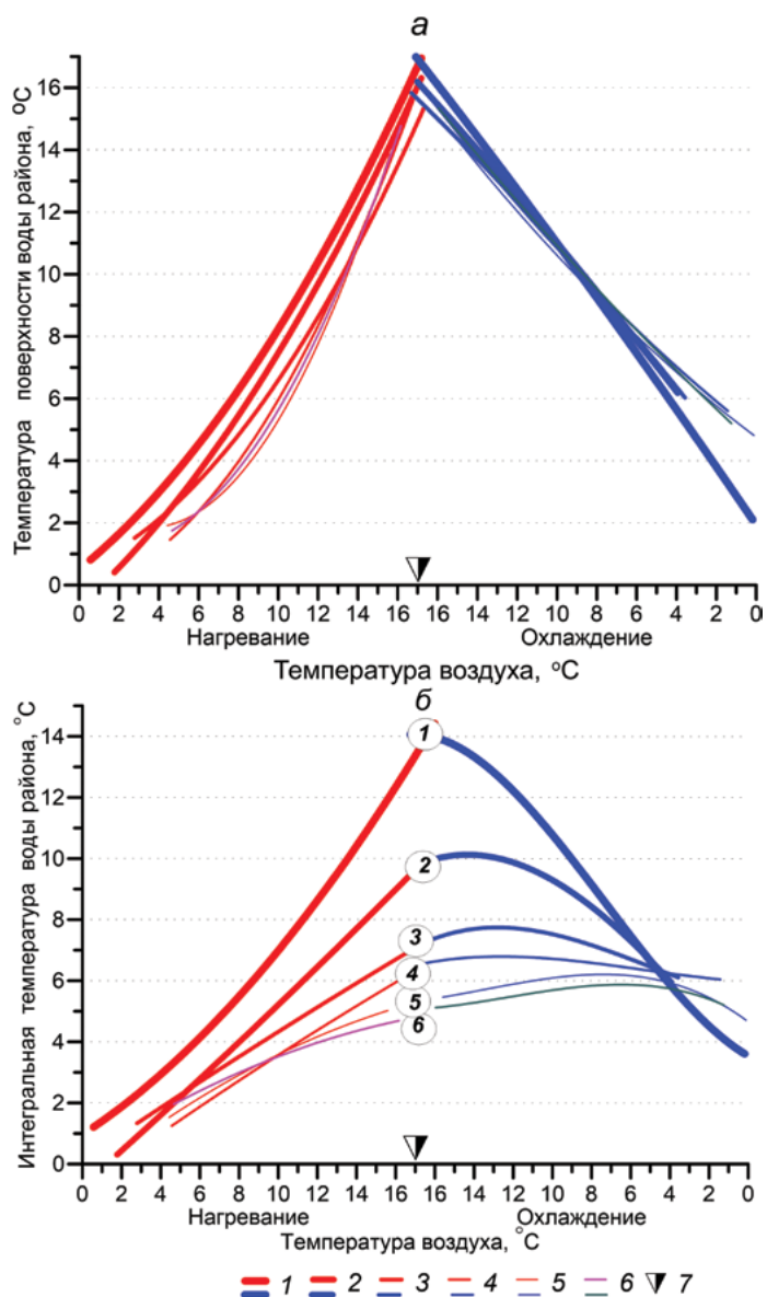
Рис. 3.5. Изменения температуры поверхности воды (а) и интегральной температуры лимнических районов Ладожского озера в зависимости от температуры приводного слоя воздуха для периода нагревания и охлаждения (б)
