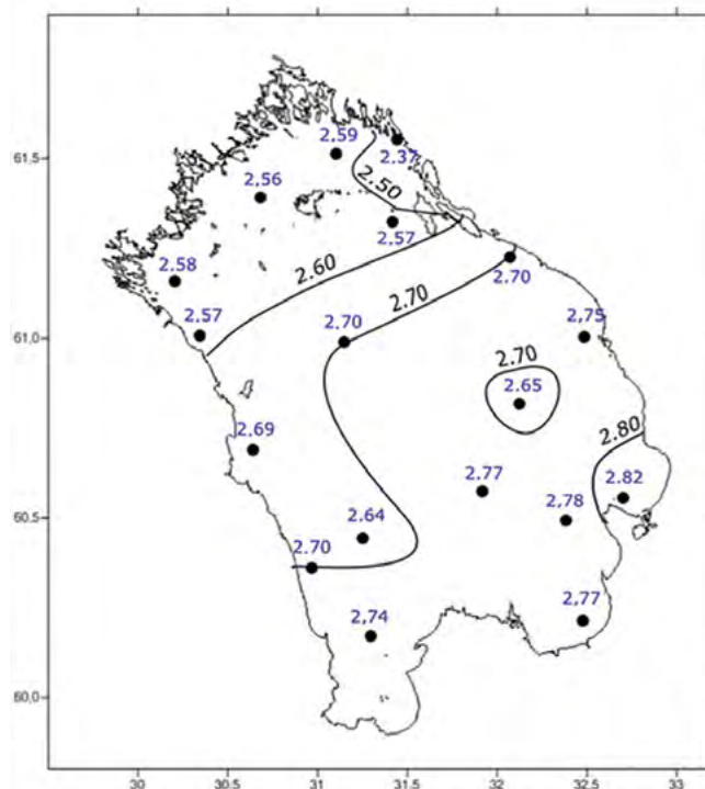
Рис. 11.10. Карта-схема распределения плотности донных отложений Ладожского озера
