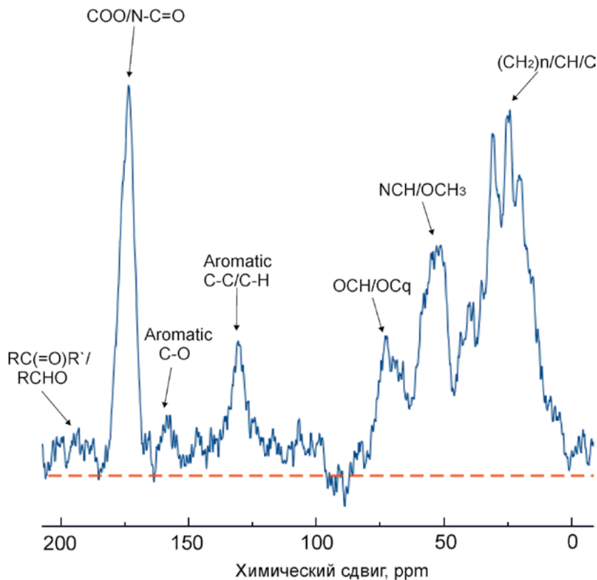
Рис. 7.7. 13С-ЯМР спектр гуминовых кислот, выделенных из донных отложений оз. Гуминового (ст. Русская, Западная Антарктида)
