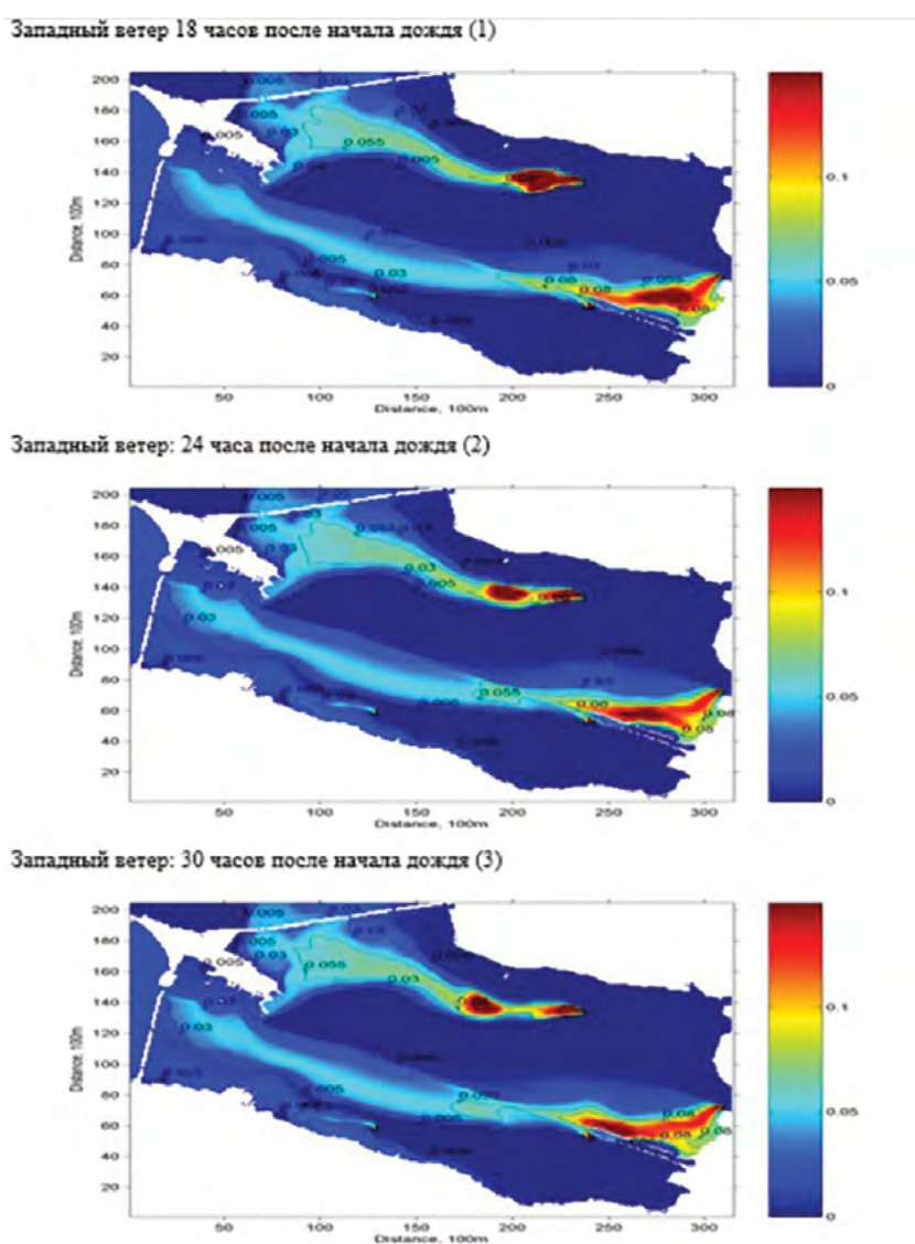
Рис. 12.5. Распределение поверхностной концентрации P_{\text{общ}} (мг/л) в Невской губе через 18(1), 24 (2) и 30 (3) часов после начала выпадения осадков. Летний стоково-ветровой режим при расходе Невы 2540 \text{ м}^3/\text{с} и западном ветре 3,5 \text{ м/с}
