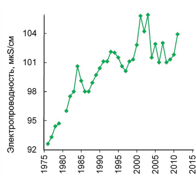
Рис. 5.12. Электропроводность воды в Ладожском озере в 1976–2015 гг.
